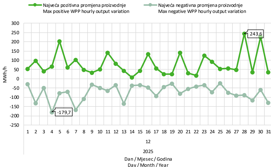
Slika 9 Maksimalna pozitivna i maksimalna negativna promjena satne proizvodnje VE u prosincu 2025. godine
