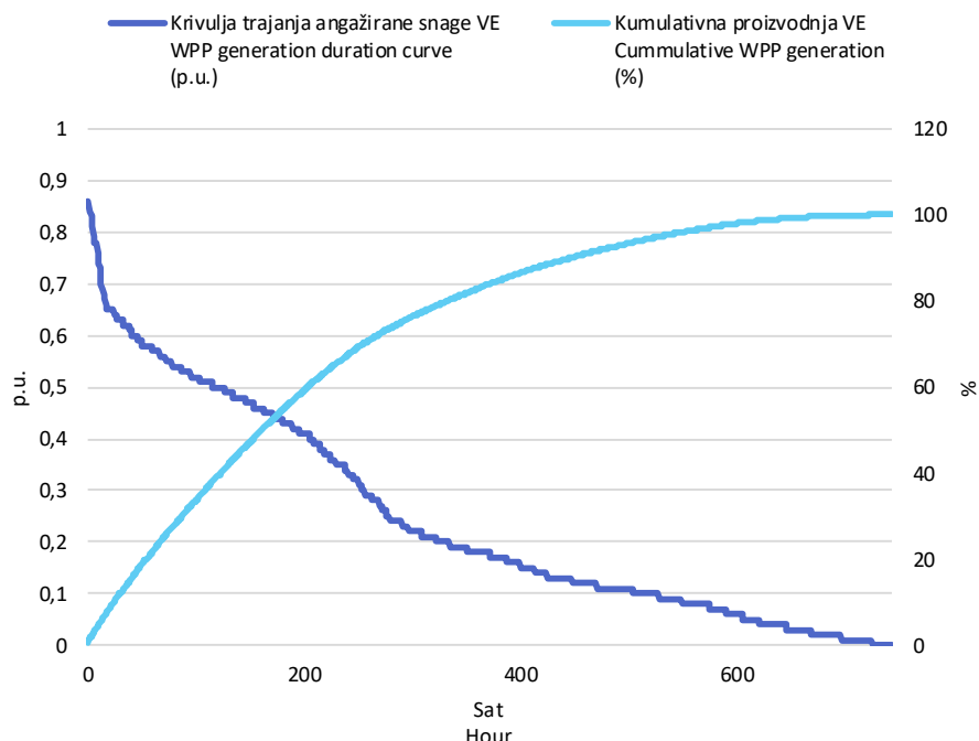
Slika 3 Krivulja trajanja angažirane snage svih VE i kumulativna proizvodnja VE u prosincu 2025. godine u jediničnim vrijednostima
