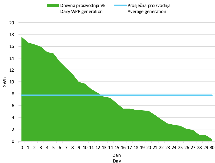
Slika 6 Krivulja trajanja dnevne proizvodnje vjetroelektrana u prosincu 2025. godine
