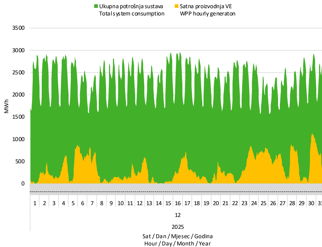
Slika 7 Usporedba satnog dijagrama opterećenja sustava i proizvodnje vjetroelektrana u prosincu 2025. godine
