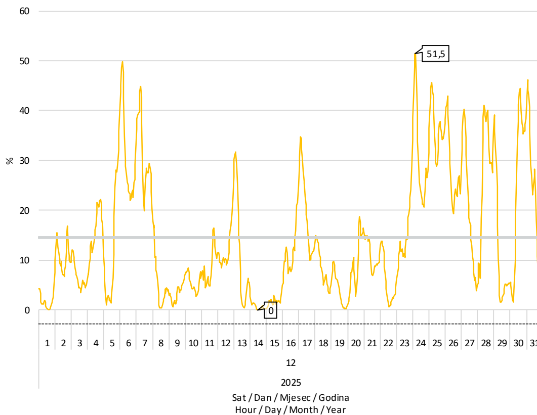
Slika 8 Udio proizvodnje vjetroelektrana u pokrivanju satnog opterećenja elektroenergetskog sustava u prosincu 2025. godine
