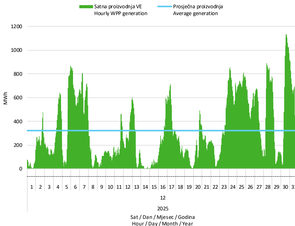
Slika 2 Satna proizvodnja svih vjetroelektrana u prosincu 2025. godine
