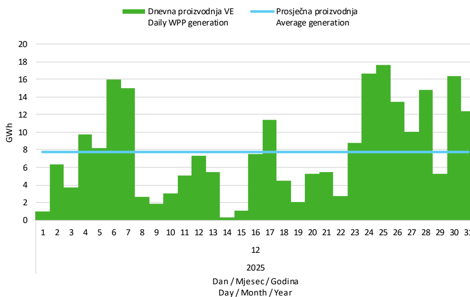
Slika 5 Dnevna proizvodnja svih vjetroelektrana u prosincu 2025. godine
