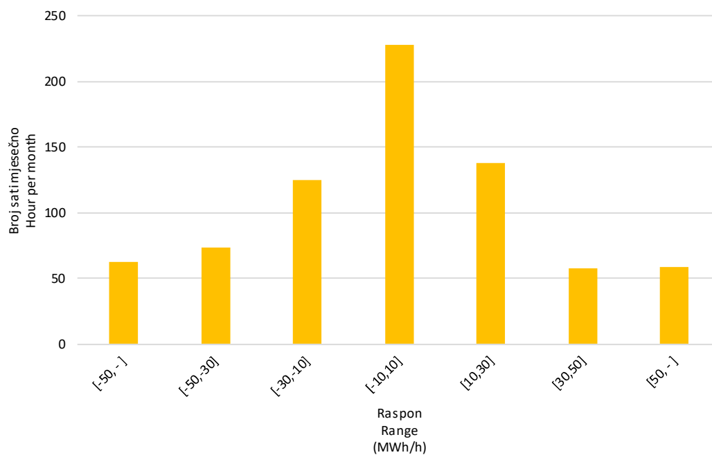
Slika 10 Statistička raspodjela satnih promjena proizvodnje VE u prosincu 2025. godine
